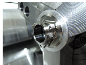
複合加工機で加工中の64チタン部品
